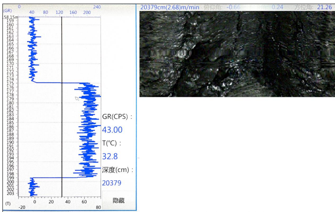
图2-7 伽马曲线
