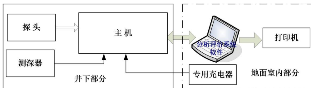
图1-2 系统组成方框图
