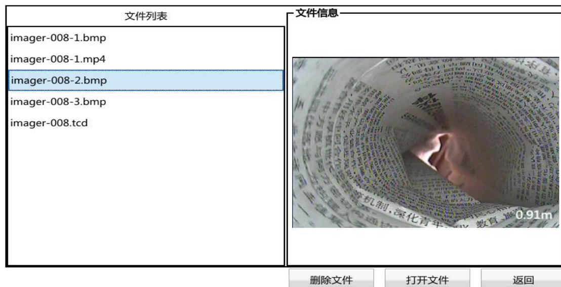
图2-9 图片浏览
