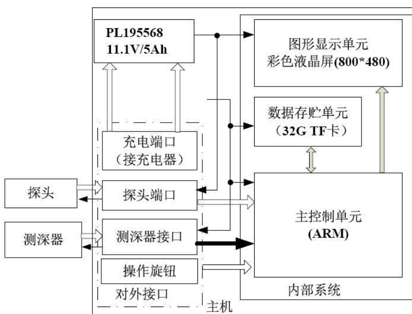
图1-3 主机结构方框图
