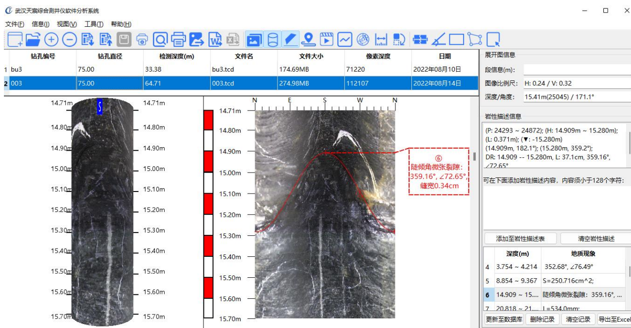
图3-10 缝宽产状图
