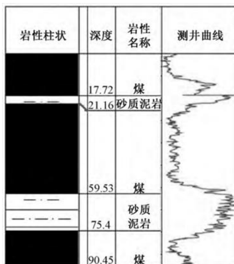
图1-4 岩性分析图
