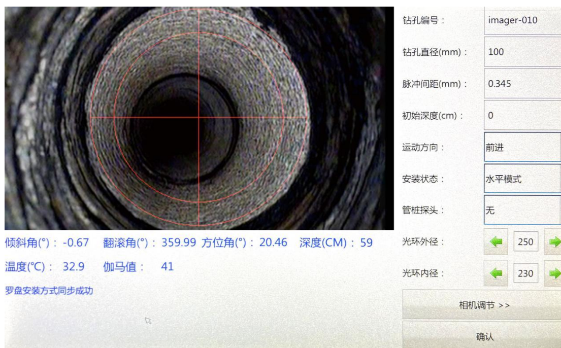
图2-5 参数设置
