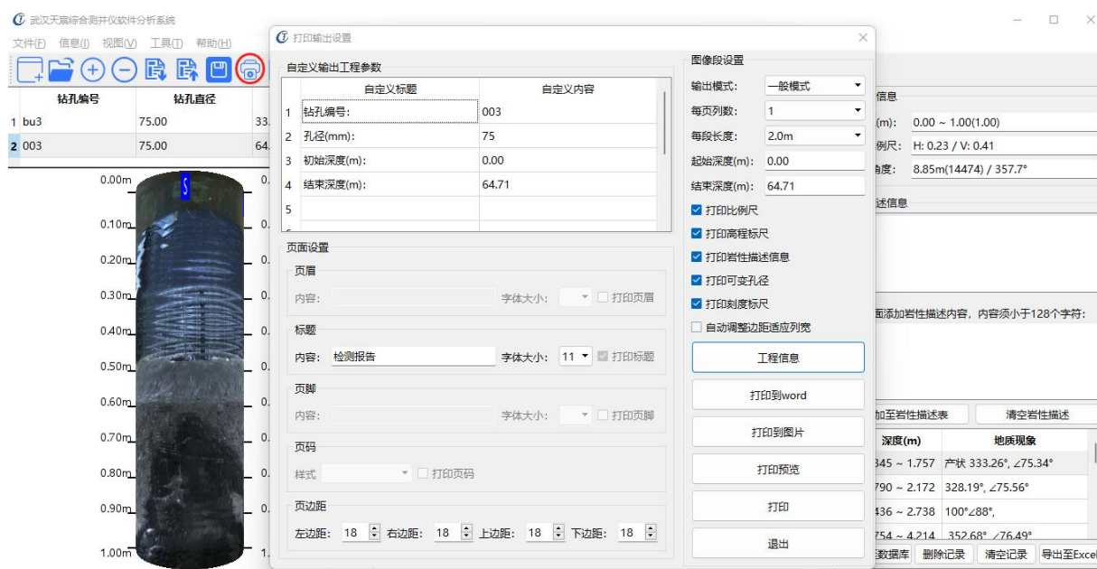
图3-22 打印设置
