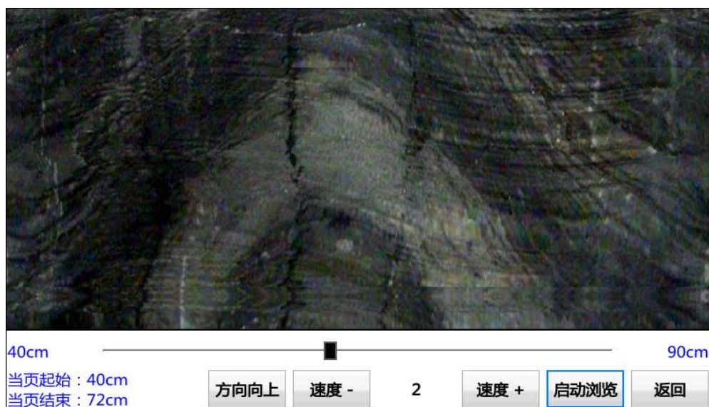
图2-11 成像浏览
