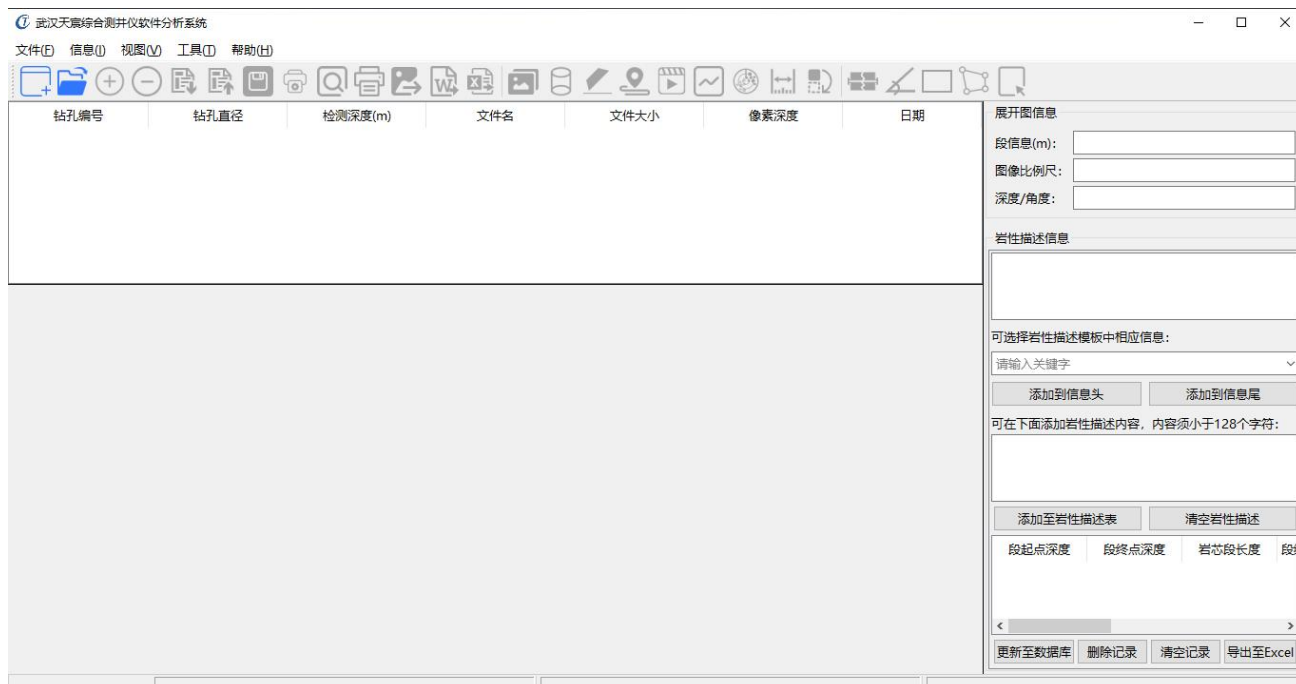
图3-2 软件主界面
