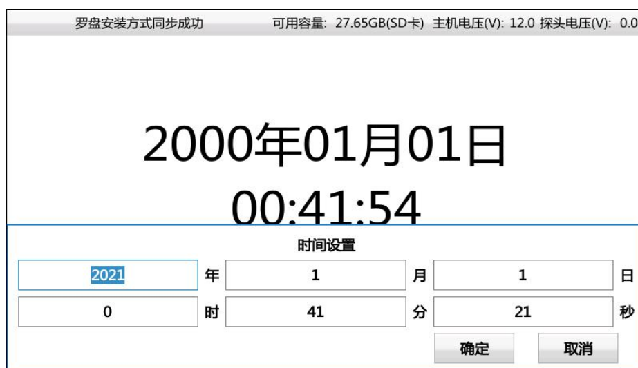
图2-12 时间校准
