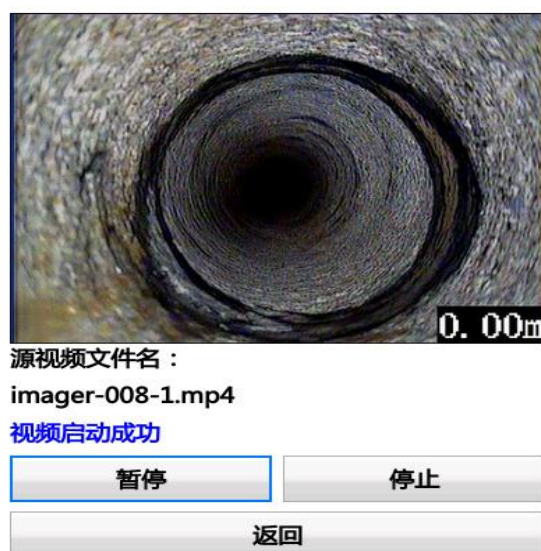
图2-10 视屏浏览
