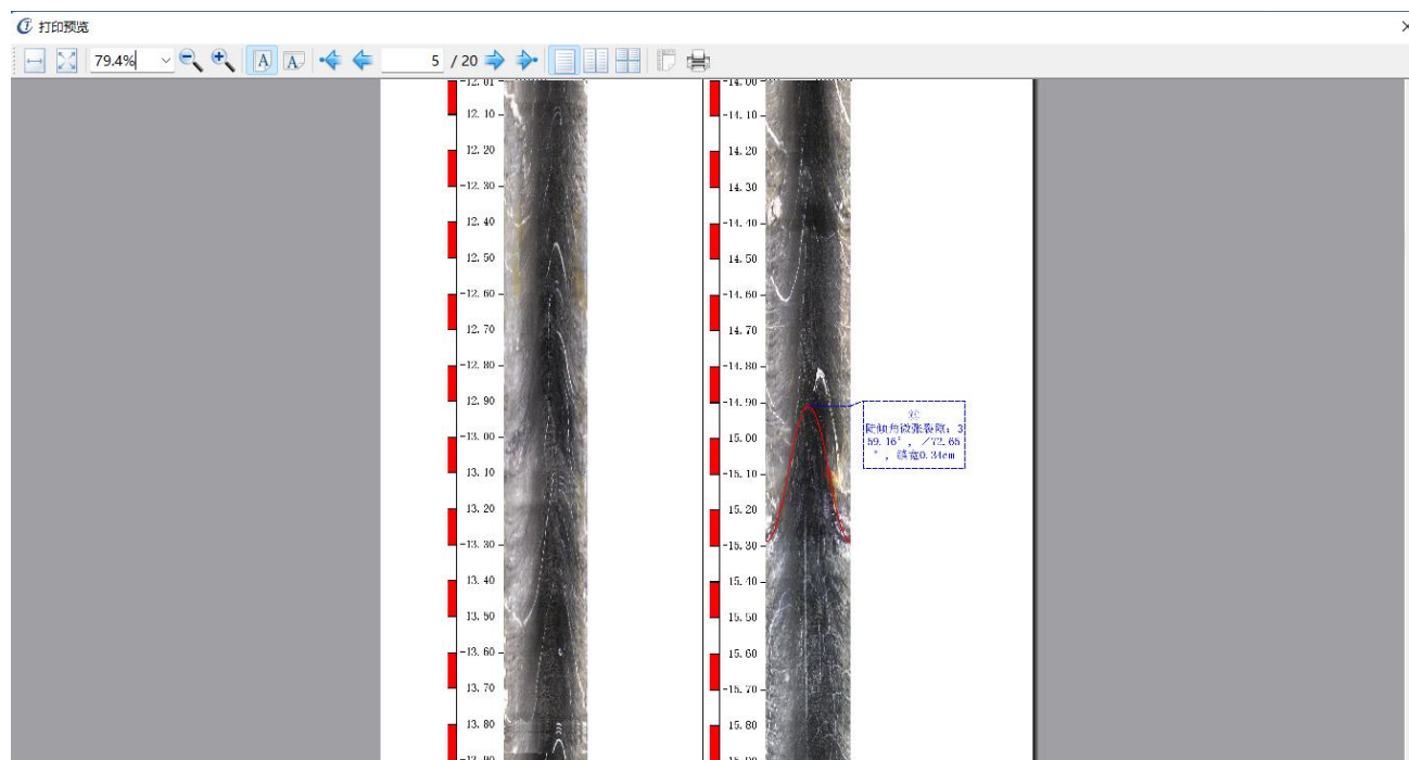
图3-28 打印预览
