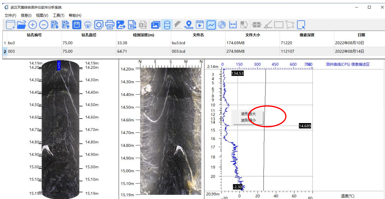
图3-15 GR曲线波形放大/缩小
