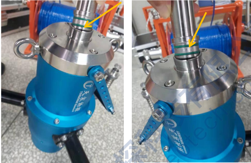
(将密封圈抹上防水硅脂，卡口对准，将插头完全插入拧紧丝扣)
