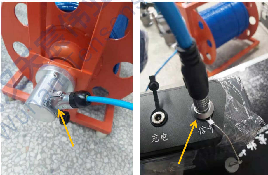
(将主机电缆连接线按图示相应连接)
