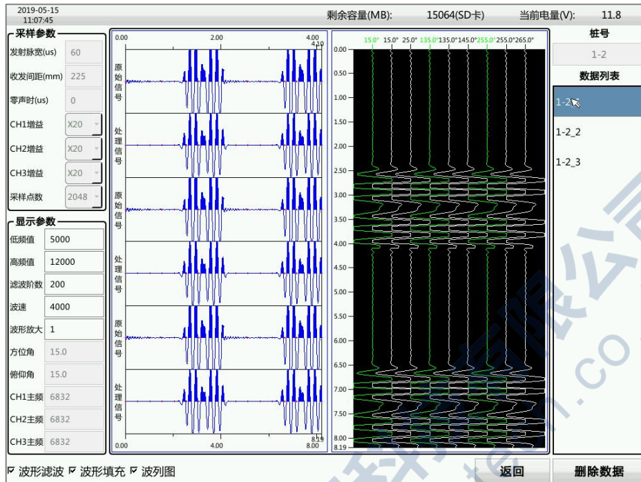
图2-12 文件浏览
