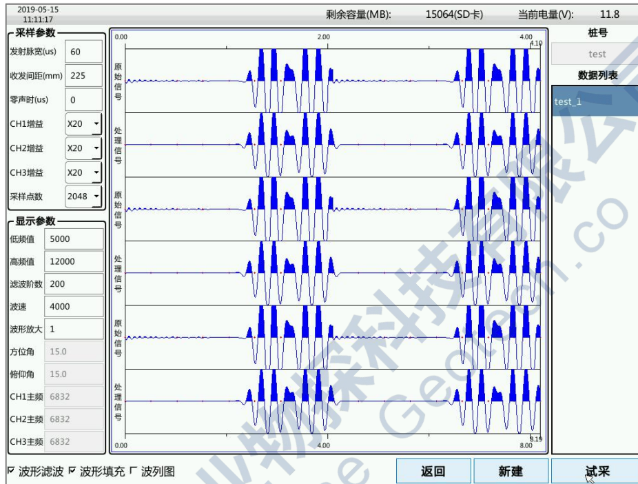
图2-5 试采界面
