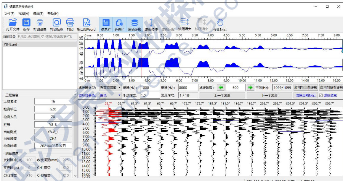
图3-9 编辑显示
